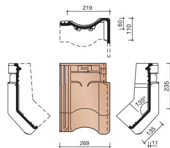
7290 RECHTER GEVELKNIKPAN
