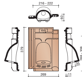
8655 MUSSENPAN
