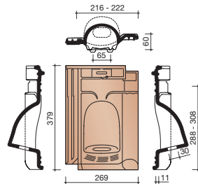
8660 GIERZWALUWPAN
