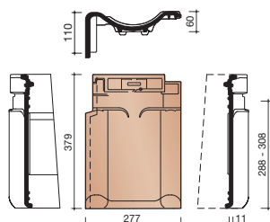
7080 LINKER GEVELPAN
