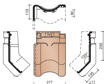
7280 LINKER GEVELKNIKPAN
