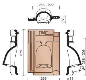
8958 KABELDOORVOERPAN
