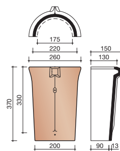
3100 SCHUBVORST
