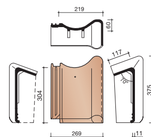
7590 RECHTER GEVELCHAPERONPAN
