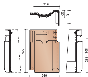
7090 RECHTER GEVELPAN
